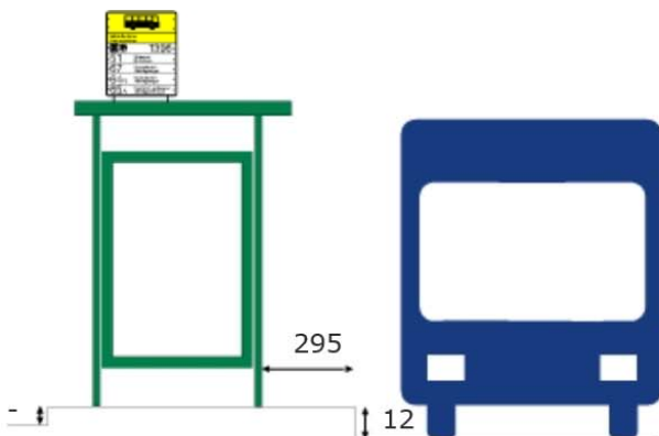
Kuva 2. Takakorotus, katoksen seinärakenteiden ja ajoradan välinen pienin etäisyys sekä pysäkin korotus ajorataan nähden. Mitat senttimetrejä.
